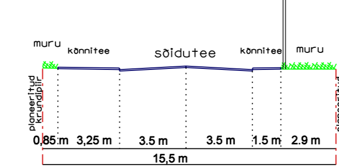
tänavaristprofiil 1:200 lõige A - A
