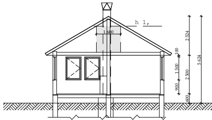
Lõige I - I M 1:100
