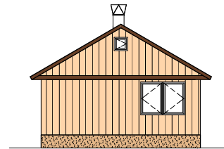
Fassaad C. M 1:100
