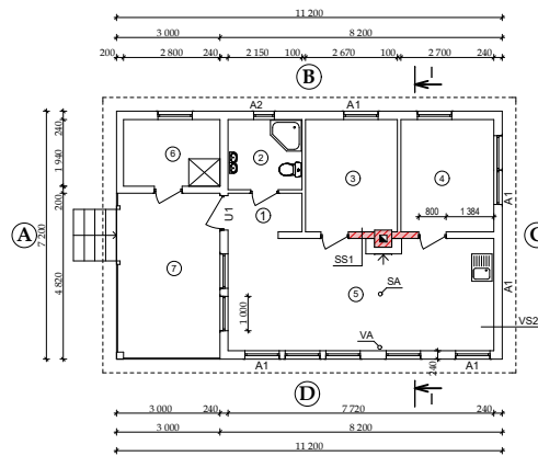
Aiamaja plaan. M 1:100
