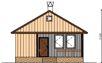
Fassaad A. M 1:100
